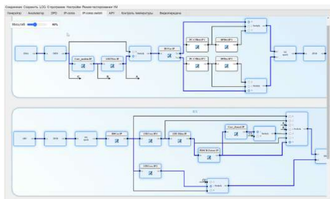
Рисунок 2 – Настройка маршрутов обработки в Signal Soft: пример расширенного FPGA-тракта
