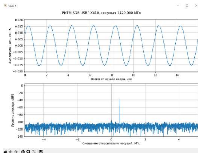
Рисунок 4 – Python/UHD: осциллограмма и спектр принятого тестового сигнала
