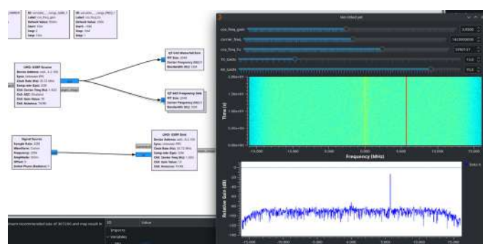
Рисунок 7 – GNU Radio: граф UHD и наблюдение принятого сигнала
