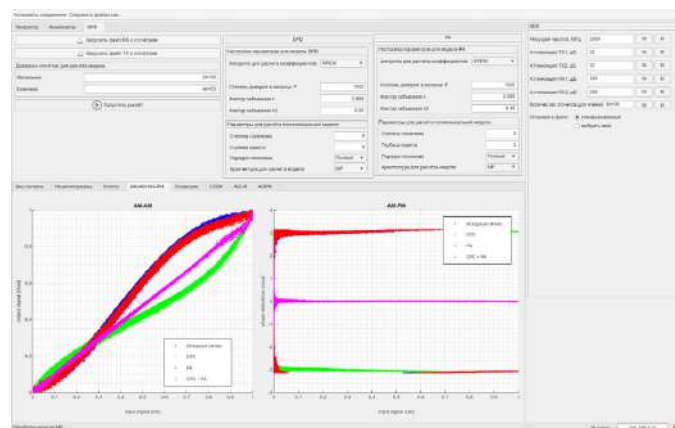
Рисунок 13 – Signal Soft: анализ характеристик AM-AM и AM-PM
