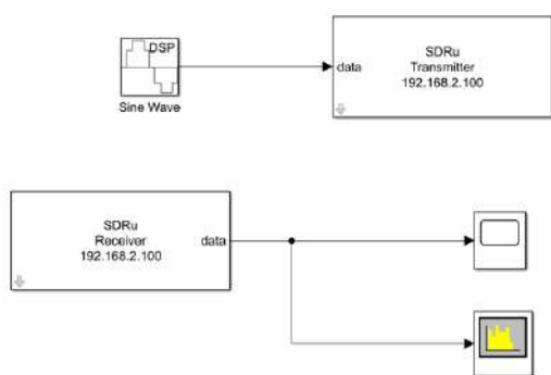
Рисунок 6 – Simulink: схема передачи и приёма с блоками SDRu
