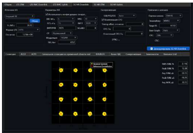
Рисунок 12 – Signal Soft: анализ созвездия и метрик 5G NR-сигнала
