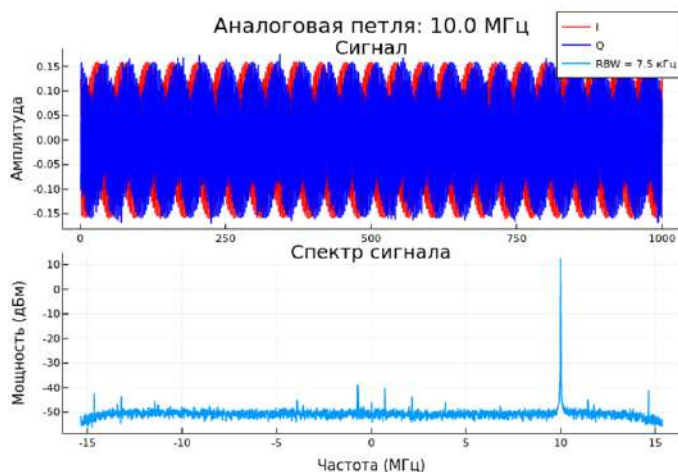
Рисунок 3 – Engee: осциллограмма и спектр принятого тестового сигнала
