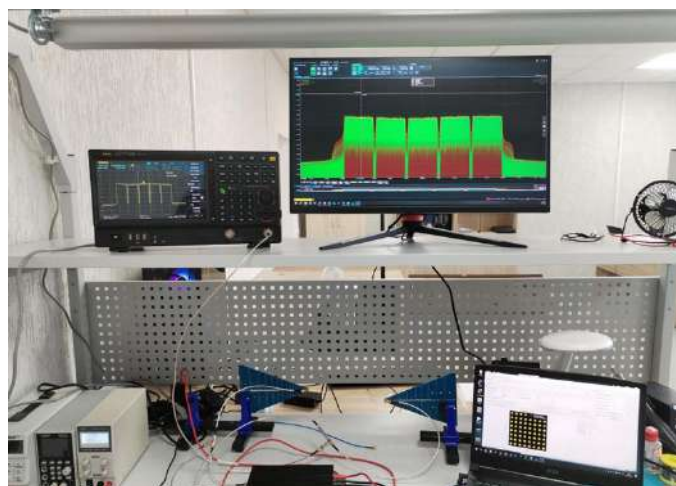
Рисунок 9 – Лабораторный стенд: наблюдение многонесущего сигнала
